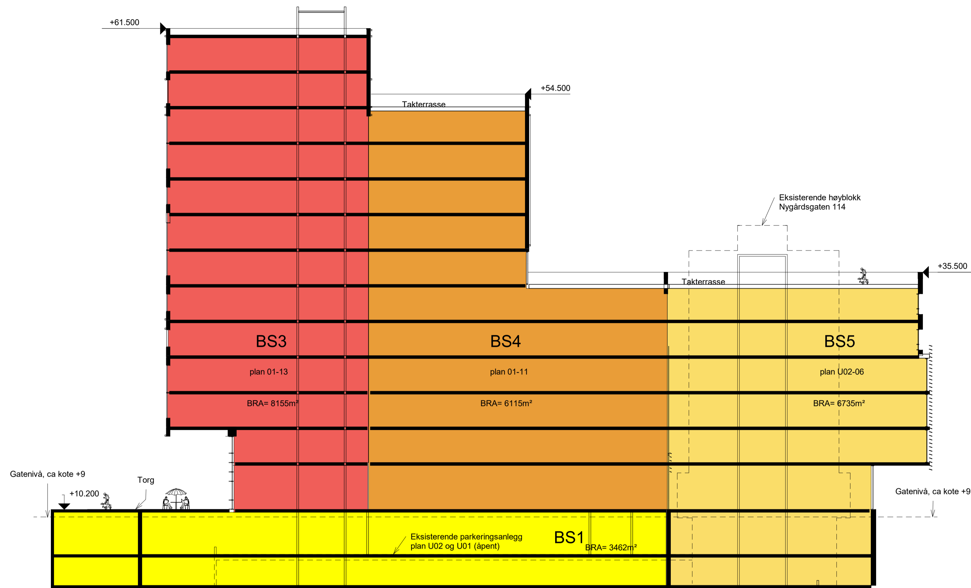
1 Snitt AA 1 : 250
