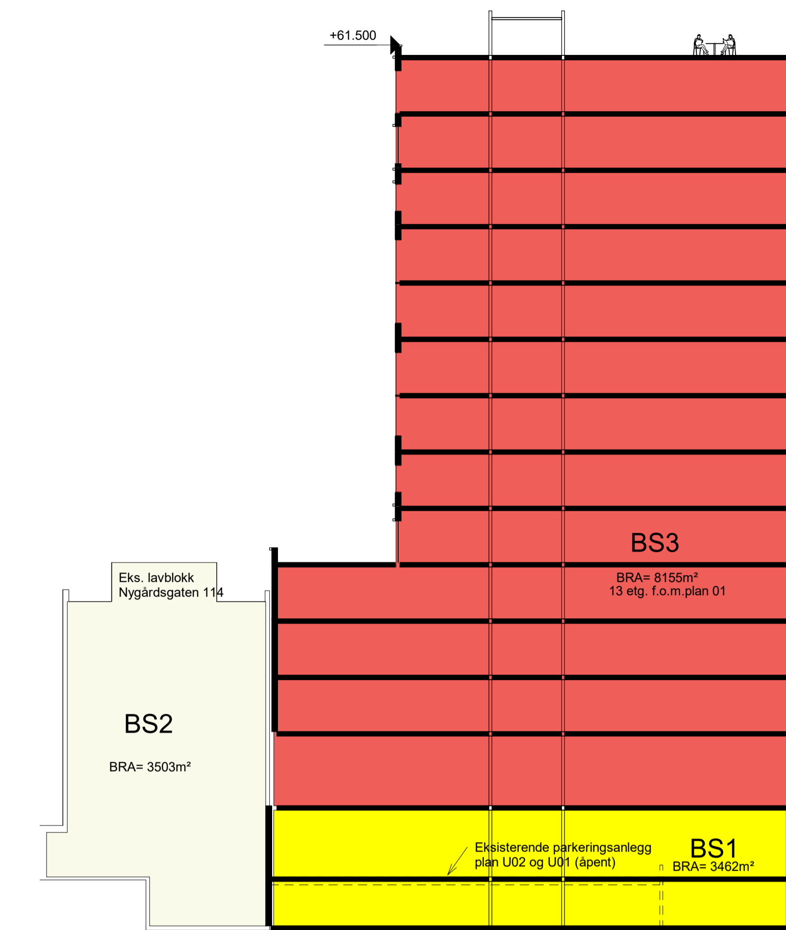
2 Snitt BB 1 : 250
